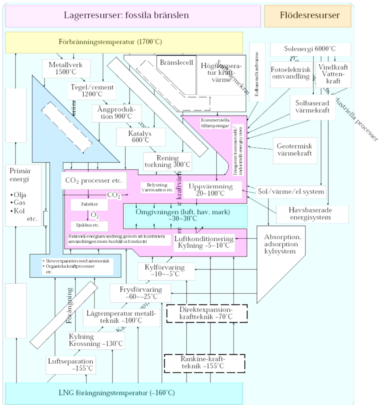
Figur 18 En integrerad resursomsättning baserad på ett högt exergiutbyte och flödesresurser.
