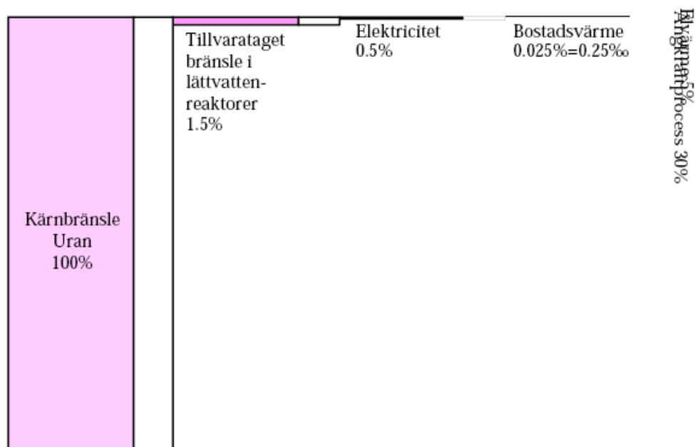
Figur 6 Utbytet för kärnkraftsproducerad el i lättvattenreaktorer för elvärme.
