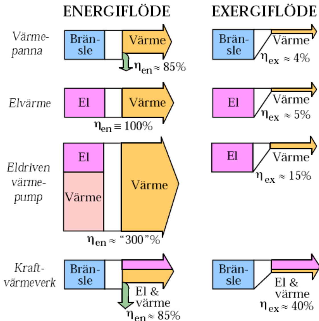
Figur 2 Energi- och exergisättningen i några energiomvandlare.
